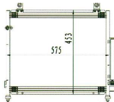
适用车型:长安之星M201 规格:575X453X16
