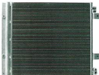
适用车型：东风天龙大力神冷凝器 芯体尺寸：580*481*20 备 注：进 5 分环保压板 / 出 3 分环保压板
