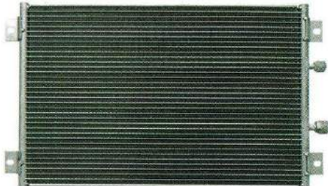
适用车型：卡特 320C 不翻边冷凝器 芯体尺寸：610*368*16 备 注：进 4 分环保外牙 / 出 3 分环保外牙
