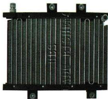
适用车型：得利卡冷凝器 芯体尺寸：295*384*32 备 注：
