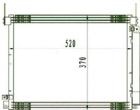
适用车型:优优(开瑞) 规格:520X370X16
