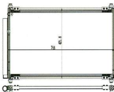
适用车型:本田奥德赛RB3 年份:09款 规格:744X422X16(波5mm) OEM:80100-SFE-003
