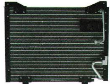
适用车型：天皇五十铃冷凝器 芯体尺寸：485*345*32 备 注：进 4 分普通压板 / 出 3 分普通端口
