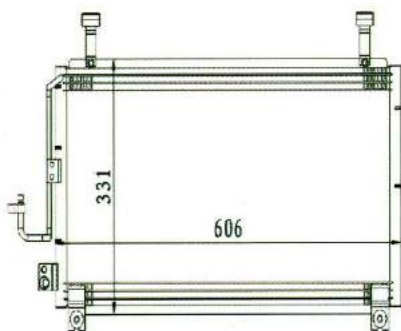
适用车型:五十铃D-MAX(东南亚)08年 规格:606X331X16
