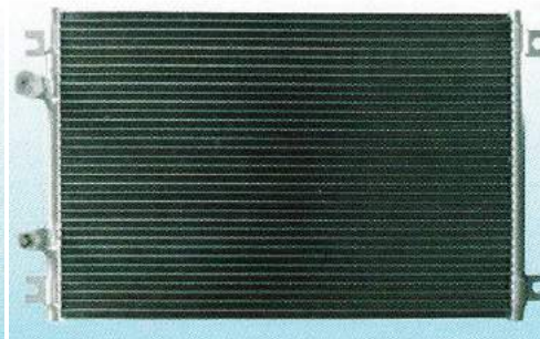
适用车型：日立 120 挖机冷凝器 芯体尺寸：583*340*20 备 注：
