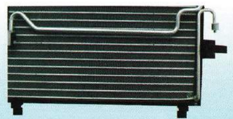
适用车型：五十铃汽油的士头冷凝器 芯体尺寸：595*345*22 备 注：进 4 分普通压板 / 出 3 分普通压嘴
