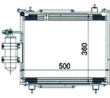
适用车型：哈飞民意冷凝器 芯体尺寸：500*360*20 备 注：进 4 分环保外牙 / 出 3 分环保端口
