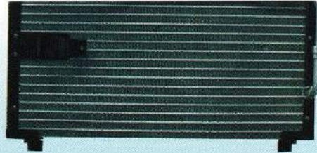
适用车型：五十铃柴油的士头冷凝器 芯体尺寸：595*345*22 备 注：进 4 分普通外牙 / 出 3 分普通外牙
