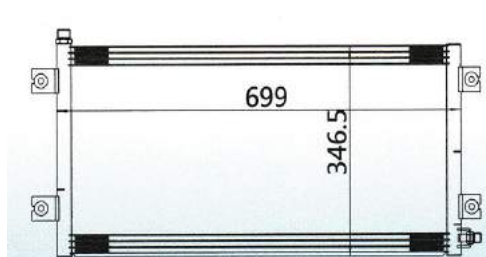
MODEL: 金王子 08 YEAR: SIZE: 699x346.5x20
