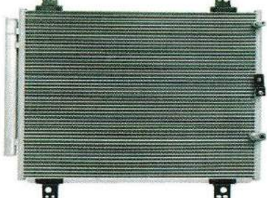
适用车型：丰田海狮冷凝器 芯体尺寸：626*506*16 备 注：
