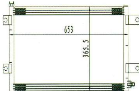
适用车型:加工金王子 规格:653X365.5X20
