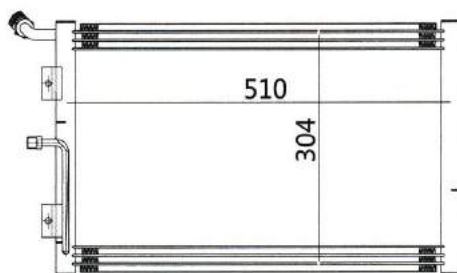
MODEL: 吉利美日 YEAR: SIZE: 510x304x20
