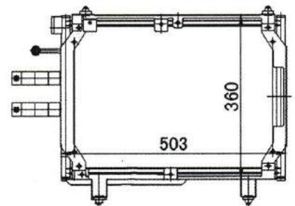
MODEL: 长安之星 (新版) YEAR: SIZE: 575x308x20
