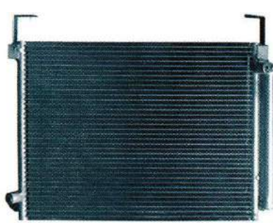
适用车型：优优（开瑞）冷凝器 芯体尺寸：520*370*16 备 注：
