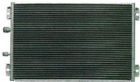
适用车型：卡特 320C 挖机冷凝器 芯体尺寸：610*368*16 备 注：进 4 分环保外牙 / 出 3 分环保外牙
