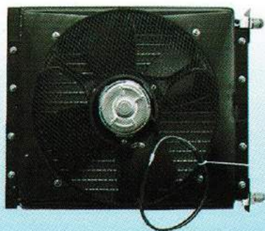
适用车型：一汽红塔冷凝器总成 芯体尺寸：470*345*32 备 注：24V/12V
