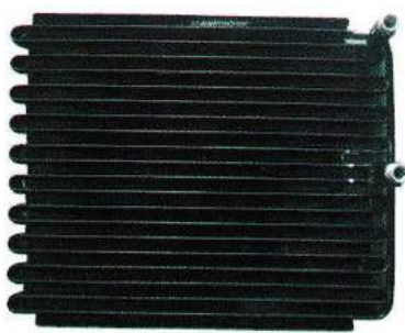
适用车型：康明斯单网冷凝器 芯体尺寸：425*333*22 备 注：进出 M20*1.5OR 接头
