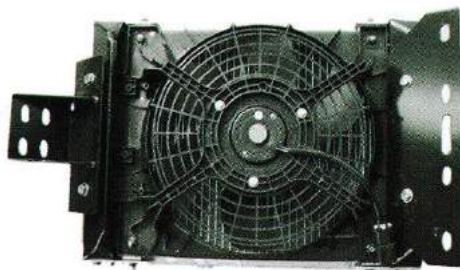
适用车型：德龙侧装冷凝器总成 芯体尺寸：488*341*20 备 注：进出 4 分环保压板
