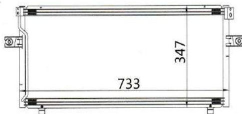
CAR MODEL: NISSAN FOISION II /ALTIMA YEAR: 93-97 SIZE: 733×347×16
