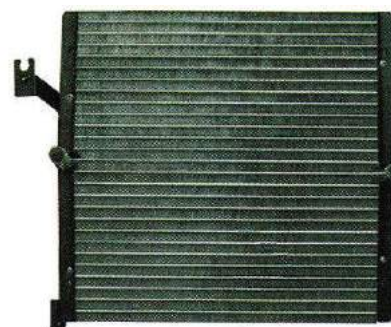
适用车型：金杯冷凝器 芯体尺寸：465*444*32 备 注：备 注：R12/R134a
