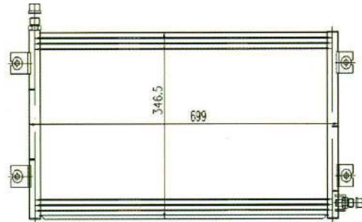
适用车型:加工网 规格:699X346.5X20
