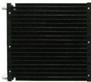
适用车型：神钢 -5 冷凝器 芯体尺寸：396*443*32 备 注：进 4 分环保外牙 / 出 3 分环保外牙
