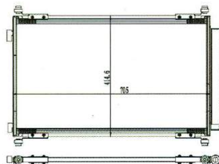
适用车型:本田讴歌MDX 年份:08款 规格:705X415X16(波5mm)
