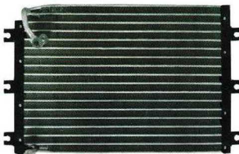
适用车型：大宇 225-7 冷凝器 芯体尺寸：557*362*26 备 注：
