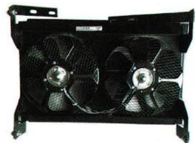
适用车型：大解放冷凝器总成 芯体尺寸：595*320*26 备 注：24V/12V
