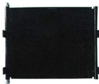
适用车型：三一重卡冷凝器 芯体尺寸：550*417*20 备 注：进 3.5 分环保外牙 / 出 3 分环保外牙
